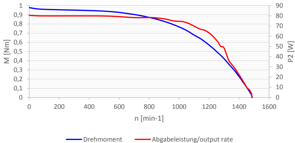
Belastungskennlinie nach IEC 60034
